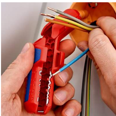
Abisolieren von Einzelleitern
