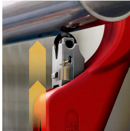
Das gefederte Schneidrad hält den KNIPEX TubiX® XL in Position und verhindert ein Verrutschen
