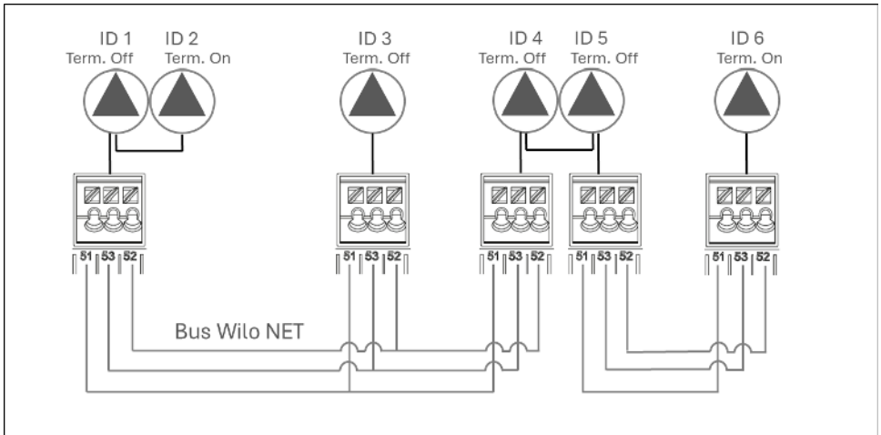
Fig. 47: Bus Wilo Net Adressierung
