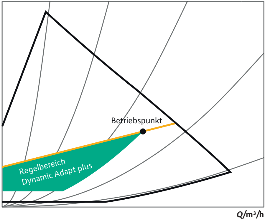
Fig. 28: Regelbereich Dynamic Adapt plus
