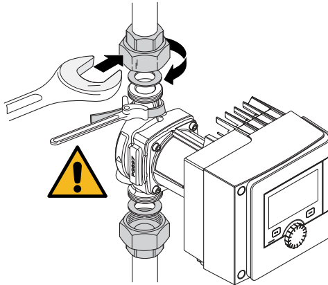
Fig. 7: Pumpe montieren
