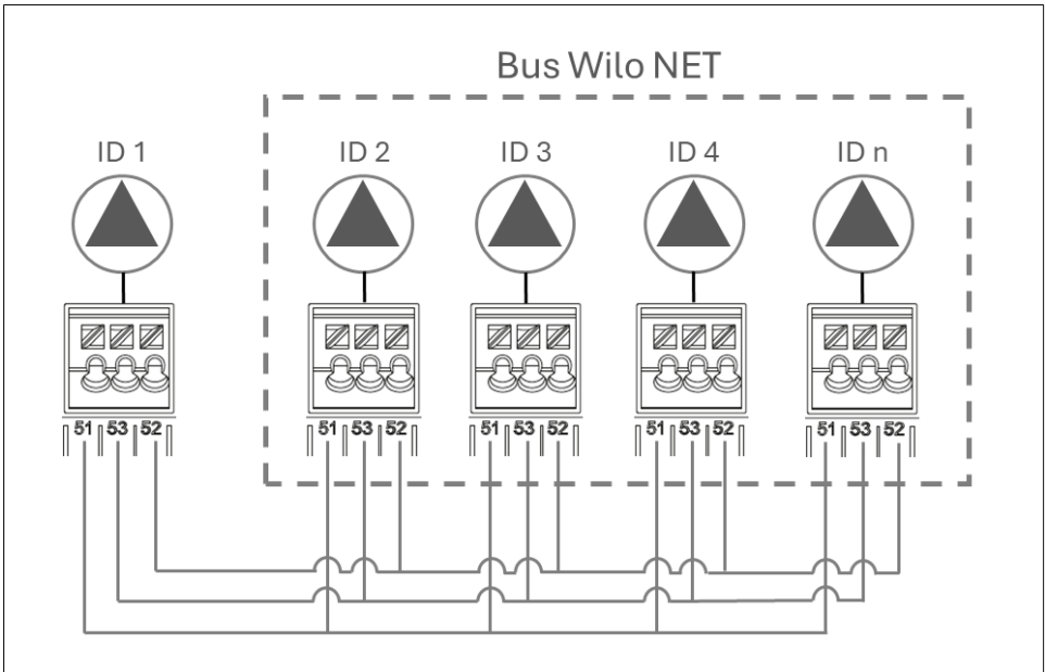
Fig. 46: Bus Wilo Net Verdrahtung
