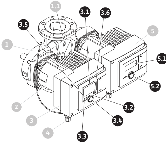
Fig. 17: Bedienelemente (Doppelpumpe)
