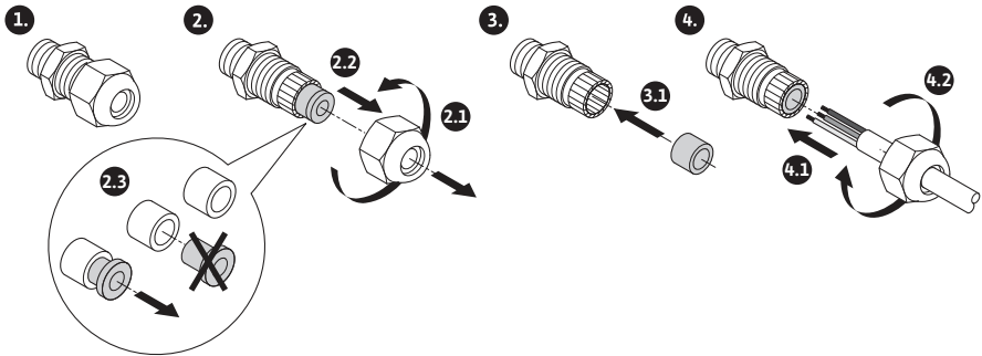
Fig. 10: Kabelverschraubung \varnothing 5 ... 10 mm
