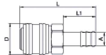
Schlauchtülle
