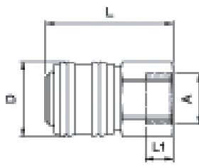
Innengewinde
