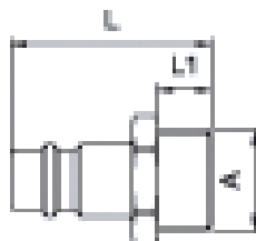
Nippel Aussengewinde
